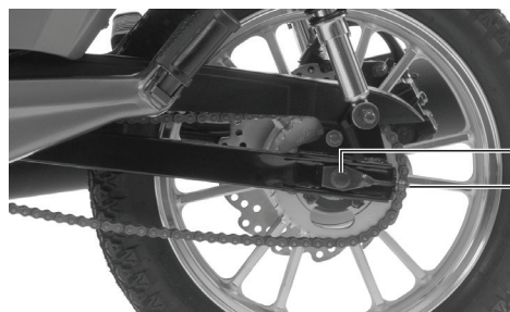
Eje de rueda trasera Tensor de cadena
